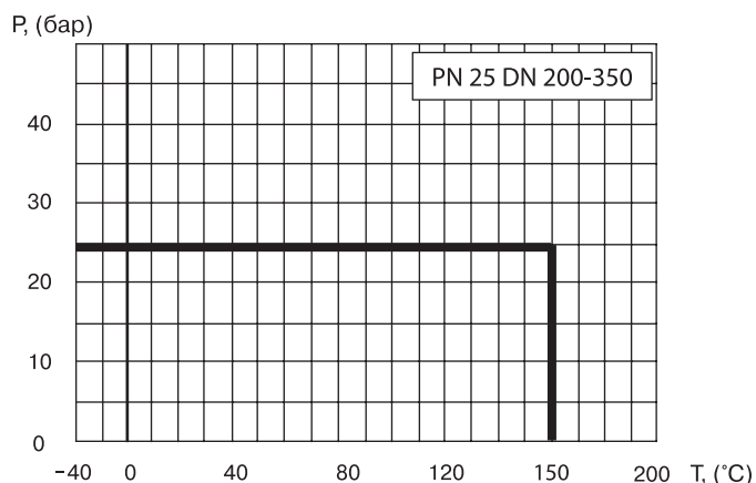
Зависимость «Температура-Давление»
