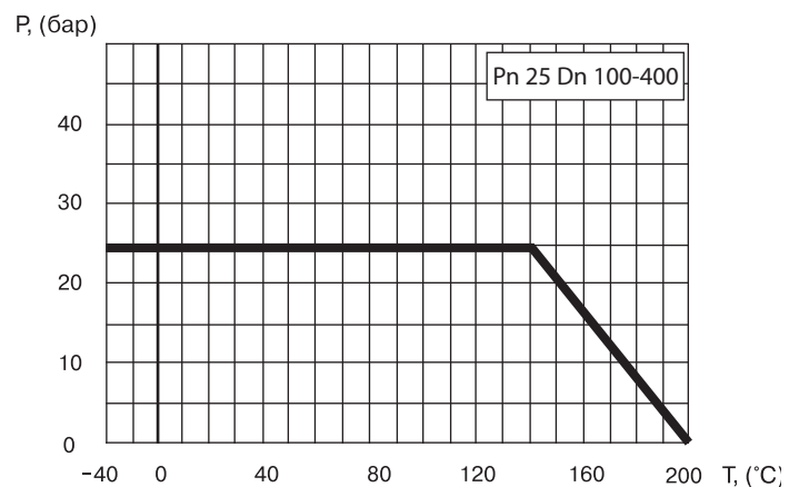
Зависимость «Температура-Давление»
