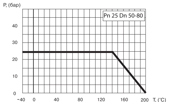
Зависимость «Температура-Давление»
