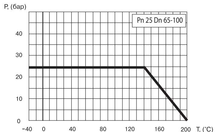
Зависимость «Температура-Давление»
